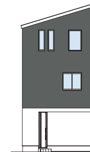
北側立面図
